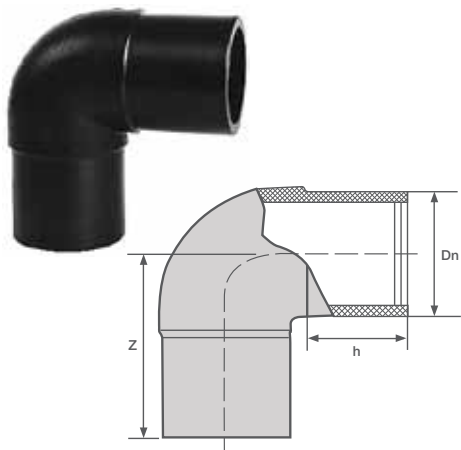
Отвод литой 90° PE 100
