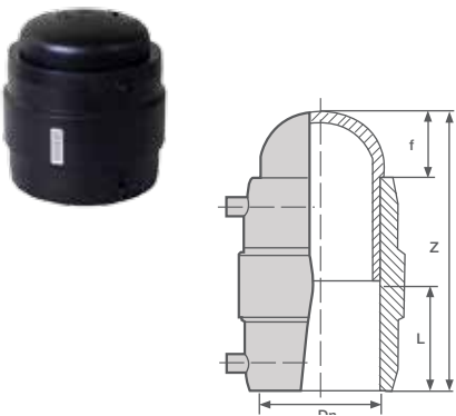
Заглушка электросварная
