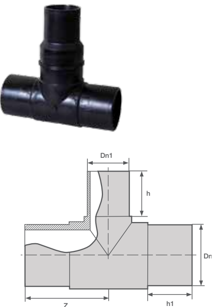
Тройник редукционный литой ПЭ100 PN10 SDR17 90° PE 100
