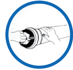
Очистить гладкий конец трубы, муфту и прокладку.
