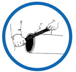
Для создания фасок ПВХ напорных труб использовать рашпиль
