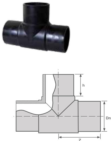
Тройник 90° PE 100
