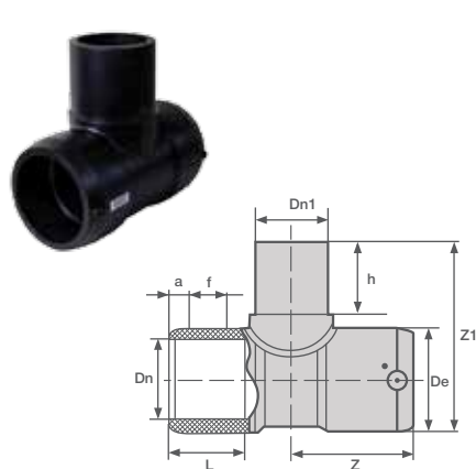
Тройник электросварной 90°
