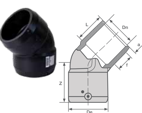
Колено электросварное 45°
