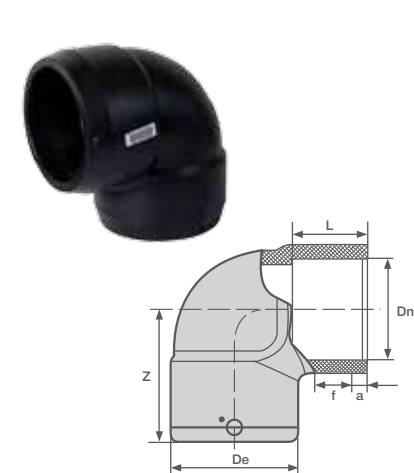
Колено электросварное 90°
